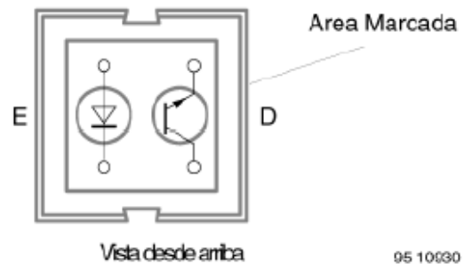
Figura 3.- Sensor CNY70
