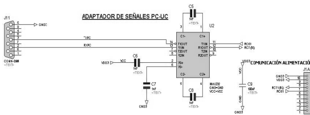
FIGURA 3. Adaptador de señales RS232/TTL
