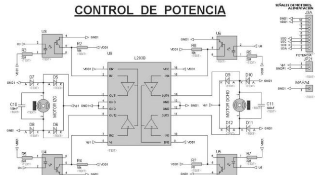
FIGURA 5. Control de potencia mediante L293
