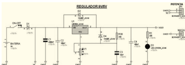
FIGURA 4. Fuente de alimentación 9V/5V.
