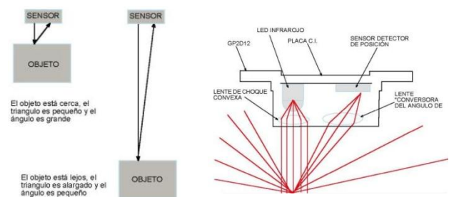
FIGURA 7. Concepto de triangulación GP2D12
