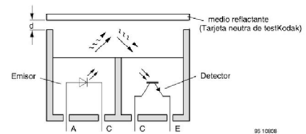
FIGURA 6. Esquema sensor infrarrojo CNY70
