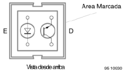
Figura 3.- Sensor CNY70
