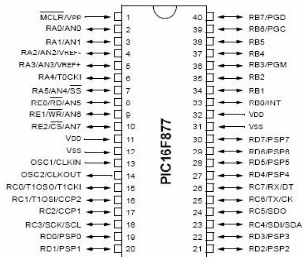
Figura 6.- Encapsulado y patinaje del PIC16F877
