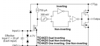
Figura 5.- Control de motores con TC4424
