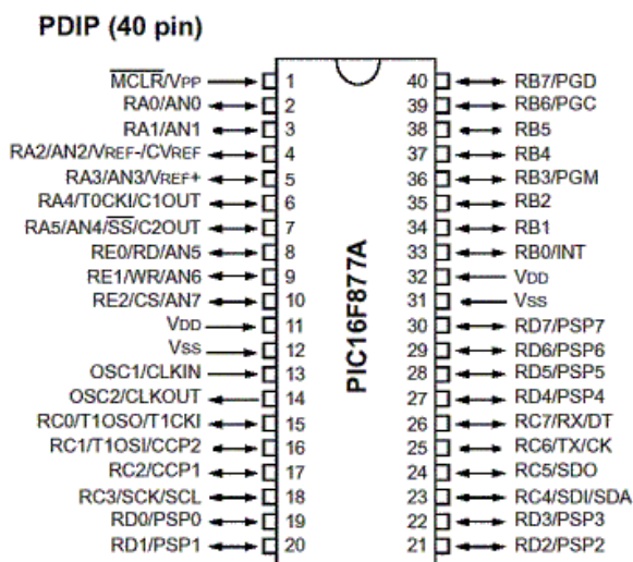
Figura 5.- Encapsulado y patillaje del PIC16F877
