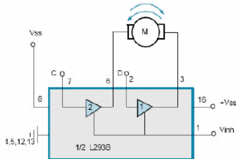
Figura 2.- Control de motores mediante L293
