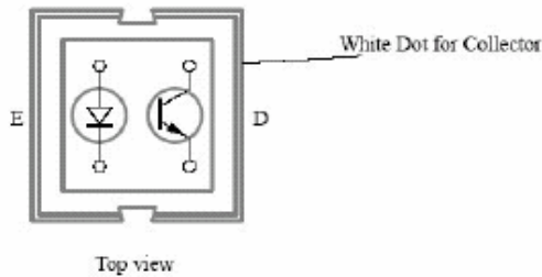
Figura 1.- Sensor CNY70
